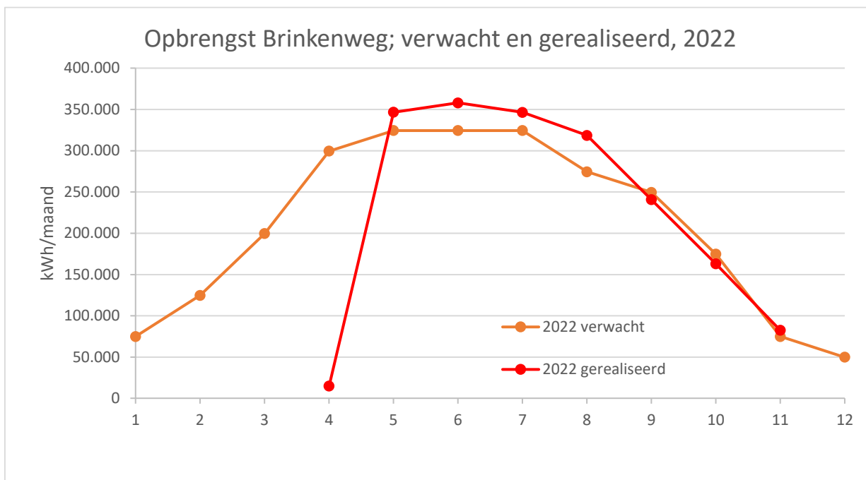
Figuur 2 Verwachte en gerealiseerde opbrengst van Zonnepark Brinkenweg (kWh/maand) voor het zonnepark in het jaar 2022 (tot november).
